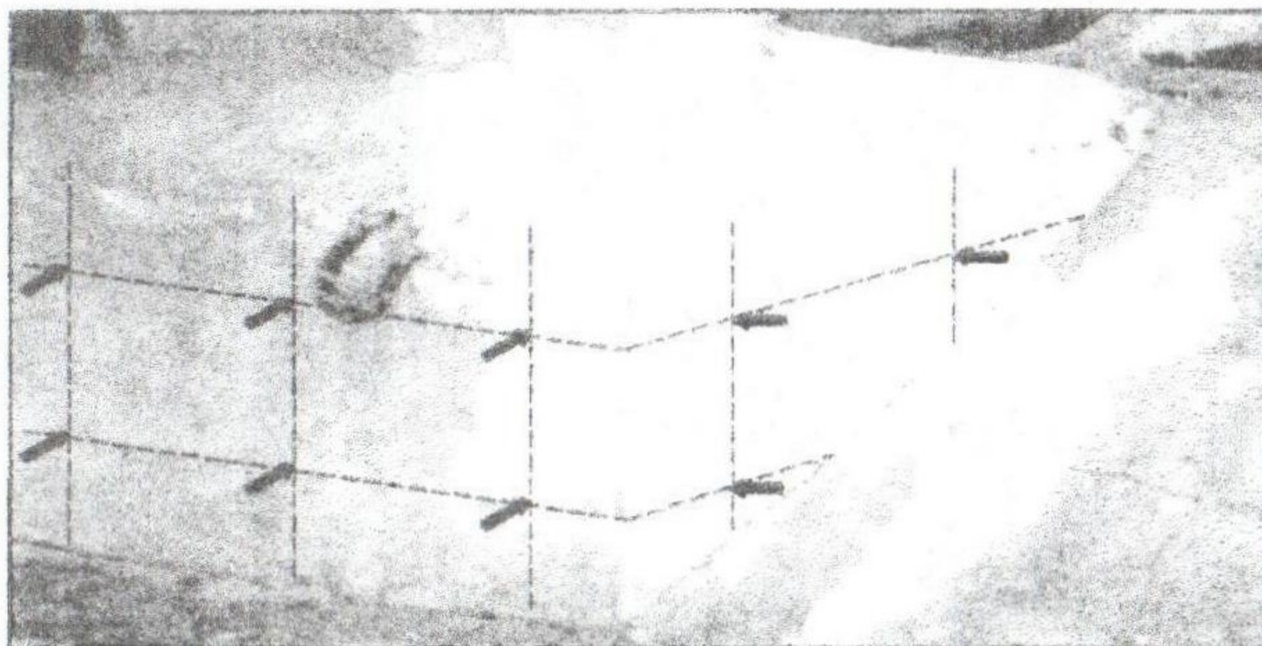
Рис. 1. Схема расположения точек возбуждения при виброакустическом контроле трехмерного объекта
