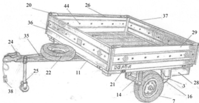
Рис 1. Конструктивна схема транспортного причепа,
