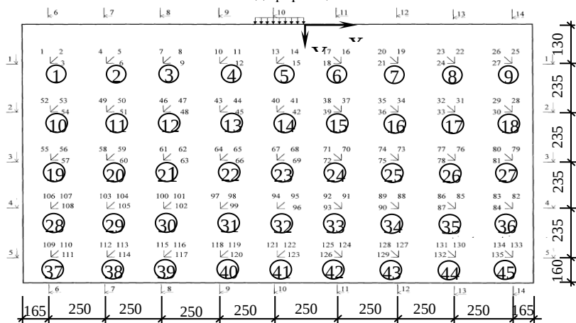
Рис.3. Схема расположения измерительных приборов на гранях столбцов: T1, T2, T3, T4, T5, T6, T11, T12, T13, T14, T15, T16 – поперечные деформации; T7, T8, T9, T10, T11, T17, T18, T19, T20, I1, I2 – продольные деформации
