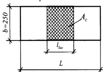
Рис.1. Нагрузка на средней части по всей ширине сечения стены
