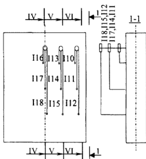
Рис.5 Схема размещения индикаторов часового типа для определения поперечных деформаций
