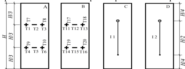
Рис.3. Схема расположения измерительных приборов на гранях столбцов: T1, T2, T3, T4, T5, T6, T11, T12, T13, T14, T15, T16 – поперечные деформации; T7, T8, T9, T10, T11, T17, T18, T19, T20, I1, I2 – продольные деформации
