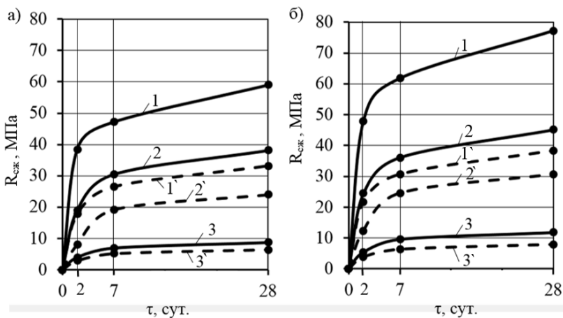
Рис. 2. Кинетика набора прочности раствора а) раствор, вяжущее которого неподвержено механоактивации; б) раствор, вяжущее которого подвержено механоактивации 1,2,3 – содержание золы-уноса в вяжущем 0, 40 и 80%, соответственно, концентрация С-3 =1%; 1',2',3' – содержание золы-уноса в вяжущем 0, 40 и 80%, соответственно, концентрация С-3 =0%
