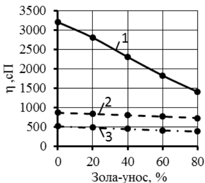
Рис. 1. Влияние добавки золы-унос на изменение эффективной вязкости цементозольной суспензии
