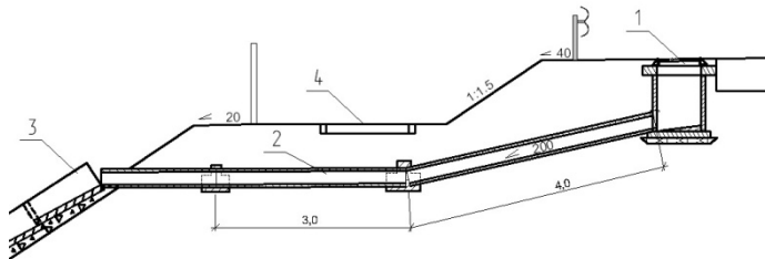
Рис. 4 Приклад застосування комбінованої системи водовідводу (а/д «Обхід м. Одеси» в межах с. Усатове): 1 – дощоприймальний колодязь; 2 – азбестоцементні труби; 3 – телескопічні лотки; 4 – тротуар
