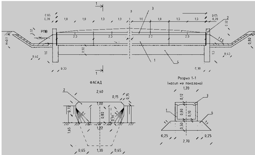
Рис 5. Конструкція закритого лотка для пропуску води під проїзною частиною 1 – середній блок; 2 – порталний оголовок; 3 – плита проїзної частини; 4 – щебенева основа
