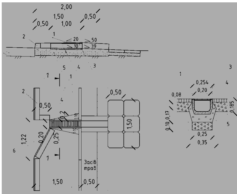
Рис. 2 Приклад застосування каналу лінійного водовідводу для скиду води під тротуаром: 1 – тротуар; 2 – бетонний борт; 3 – захисна решітка; 4 – канал лінійного водовідводу; 5 – бетонна основа; 6 – монолітний бетон водоприймальної частини
