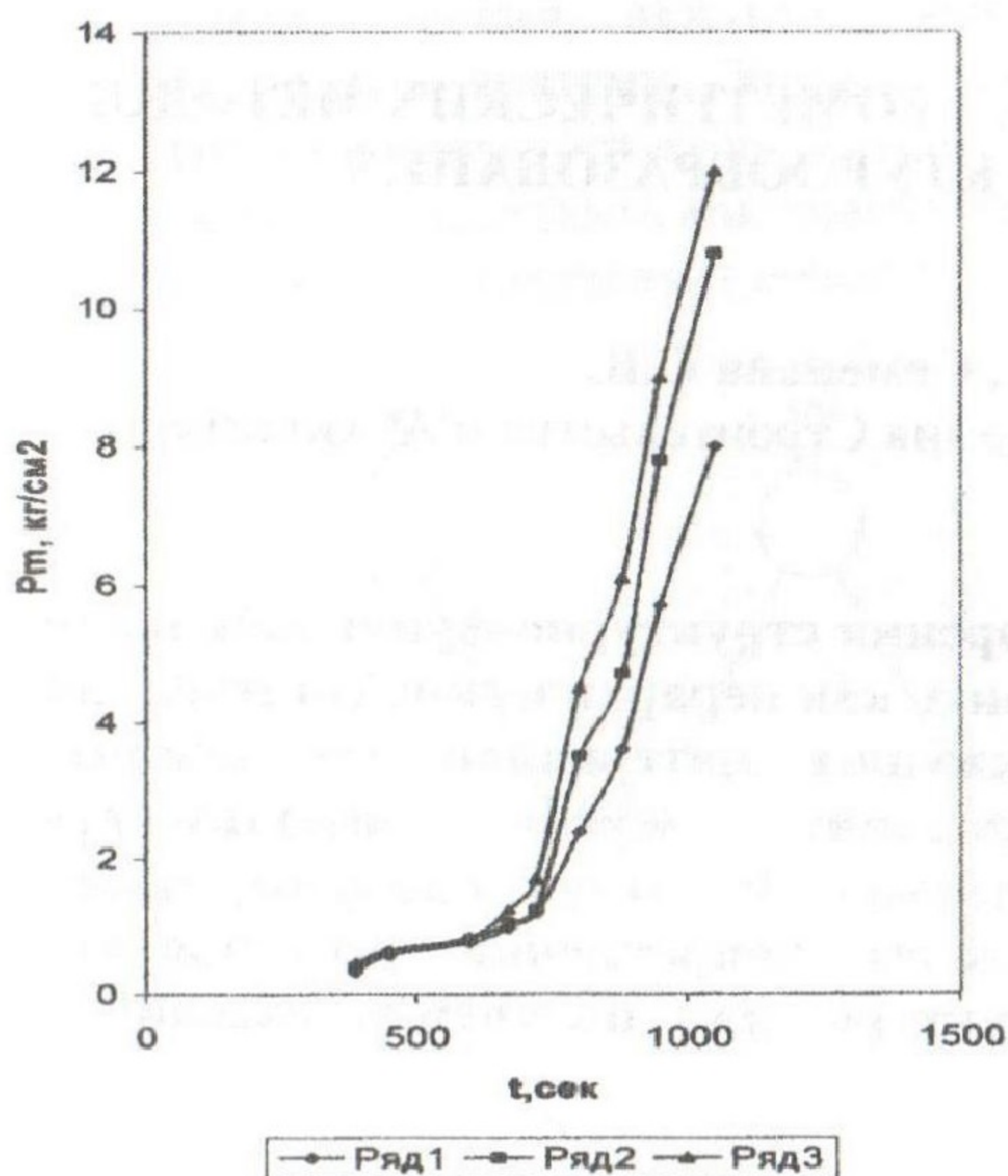
Рис. 1. Пластическая прочность гипсового теста с различной концентрацией добавки ПВС: ряд 1 – вода, C = 0 ; ряд 2 – C = 5 \text{ мг/мл} ; ряд 3 – C = 10 \text{ мг/мл} .
