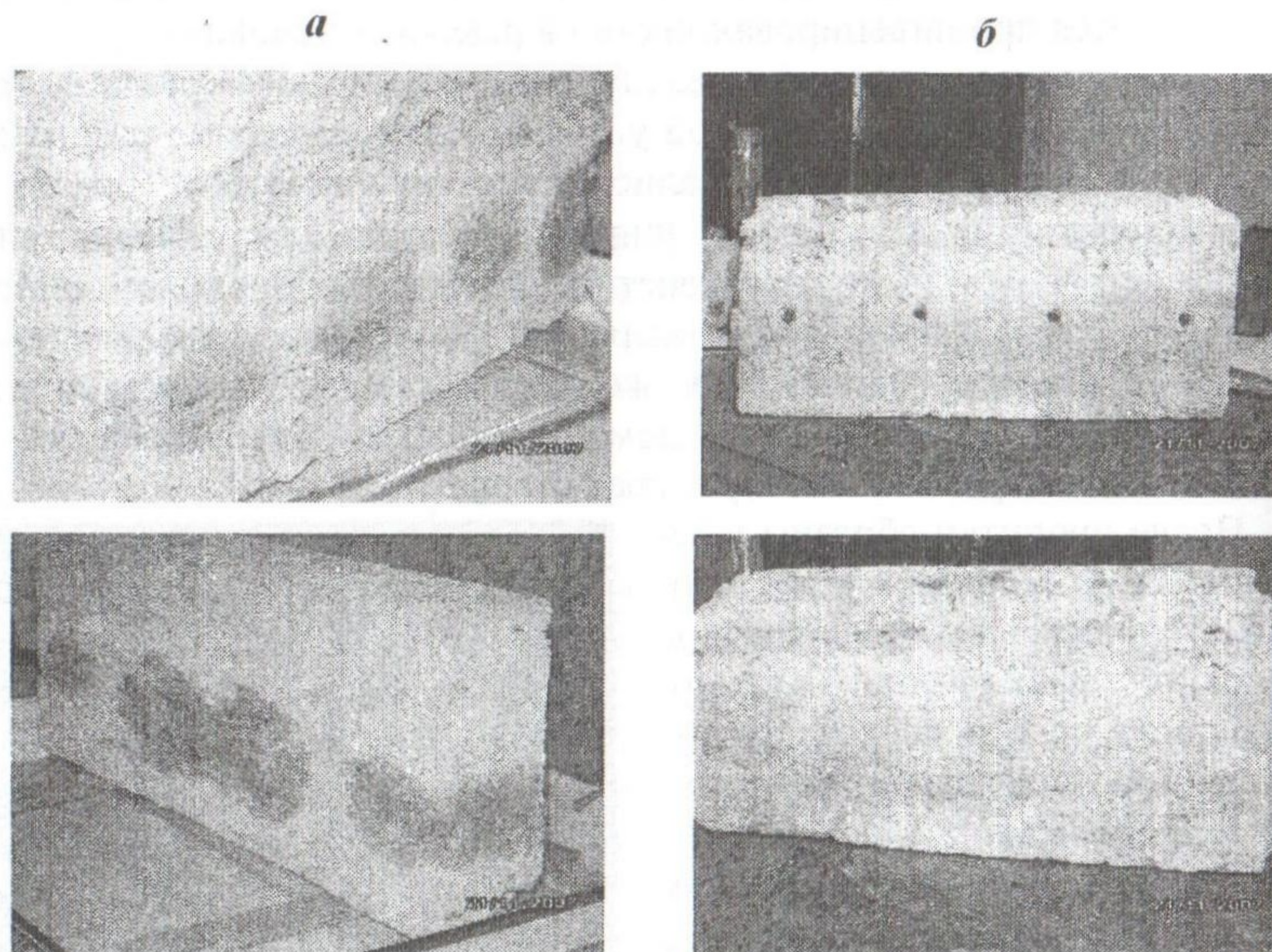
Рис.2. Определение минимального (а) и максимального (б) количества гидрофобного состава для пропитки образцов.
