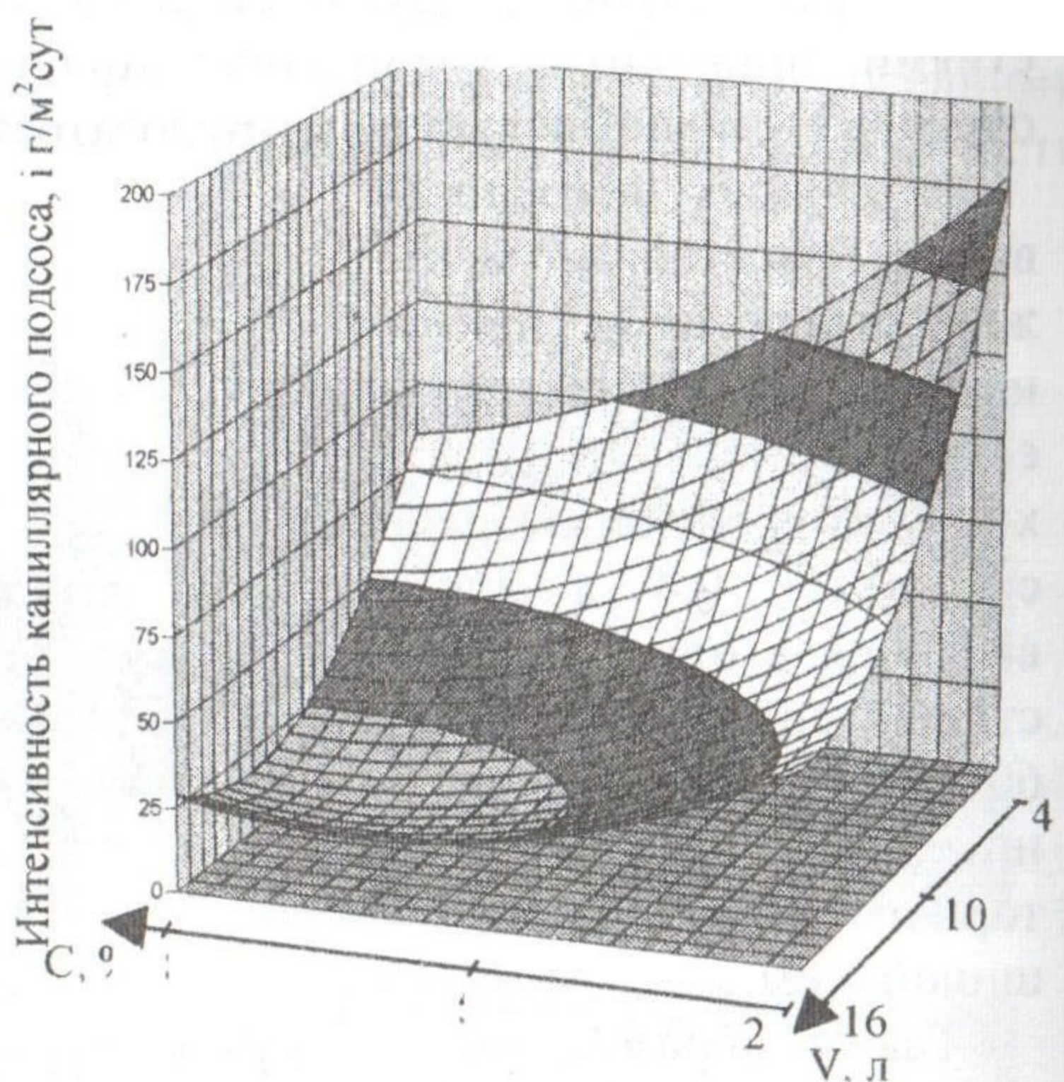
Рис. 4. Влияние расхода гидрофобного состава и его концентрации на интенсивность капиллярного подсоса
