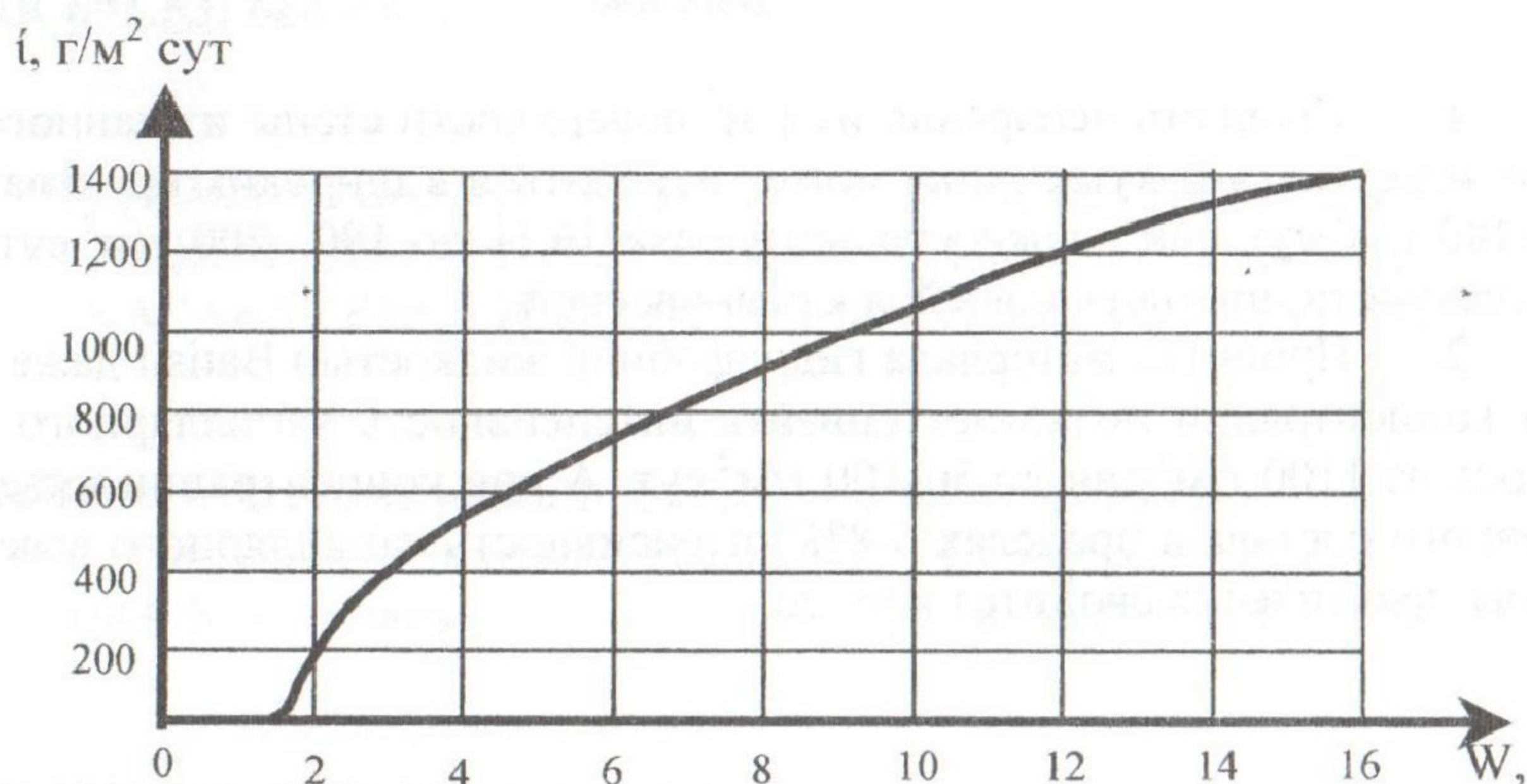
Рис.5. Влияние влажности материала стен на скорость испарения воды при температуре окружающего воздуха 18-20 °С и относительной влажности 65-70%.
