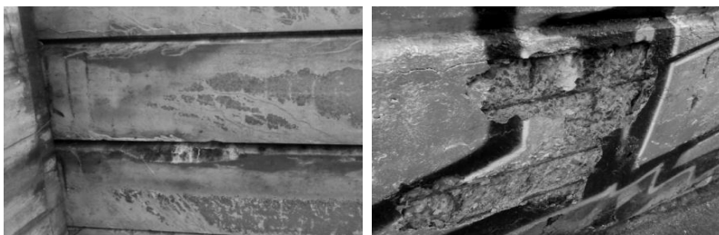
Рис.4. Мост Строганова. Сколы, отслаивание бетона, коррозия арматуры
