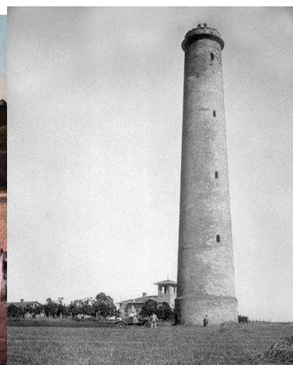
Рис. 2. Башня Ковалевского
