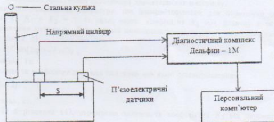
Рис. 1. Схема вимірювання швидкості пружної хвилі: S – база прозвучування
