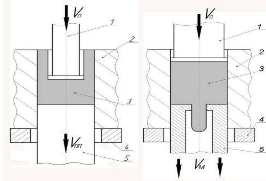
Рисунок 1. Схеми зворотного видавлювання полого виробу (а) і пресування прутка (б) з активною дією сил тертя: 1 - пуансон; 2 - контейнер; 3 - заготовка; 4 - плита; 5 - протипуансон; 6 - матриця
