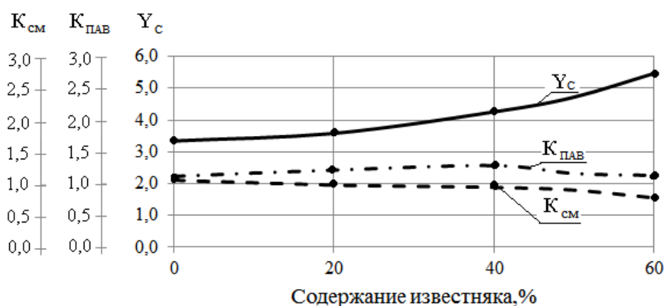
Рис. 1 Влияние количества молотого известняка на показатели Y_c , K_{см} , K_{ПАВ} - уровень синергизма Y_c ; - коэффициент K_{см} ; - коэффициент K_{ПАВ}
