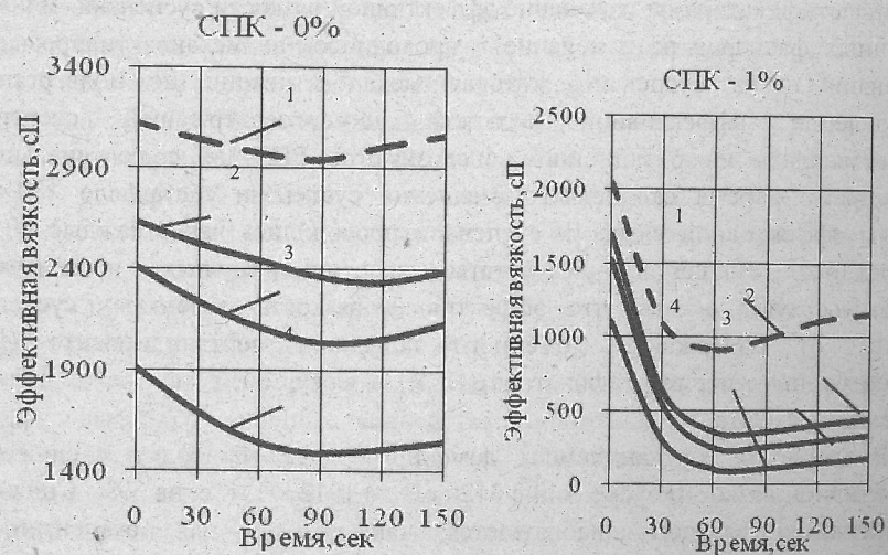
Рис 1. Влияние времени механоактивации на изменение эффективной вязкости цементосодержащей суспензии:
