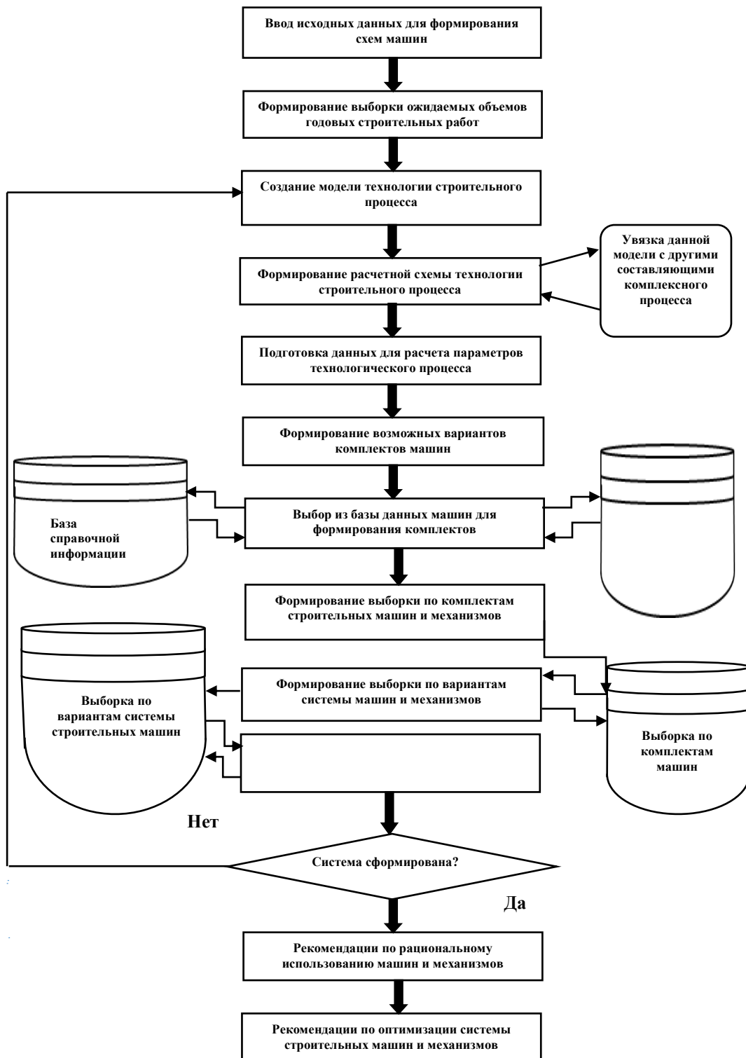
Рис. 1. Общая схема формирования систем строительных машин
