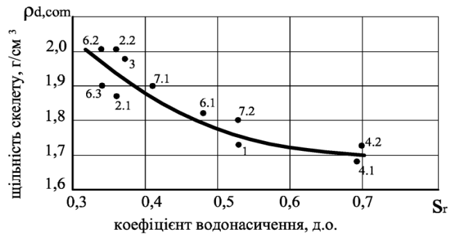
Рис.2. Залежність максимального значення щільності скелету ущільненого ґрунту від коефіцієнту його водонасичення. Цифрами показані індекси із таблиці 1.
