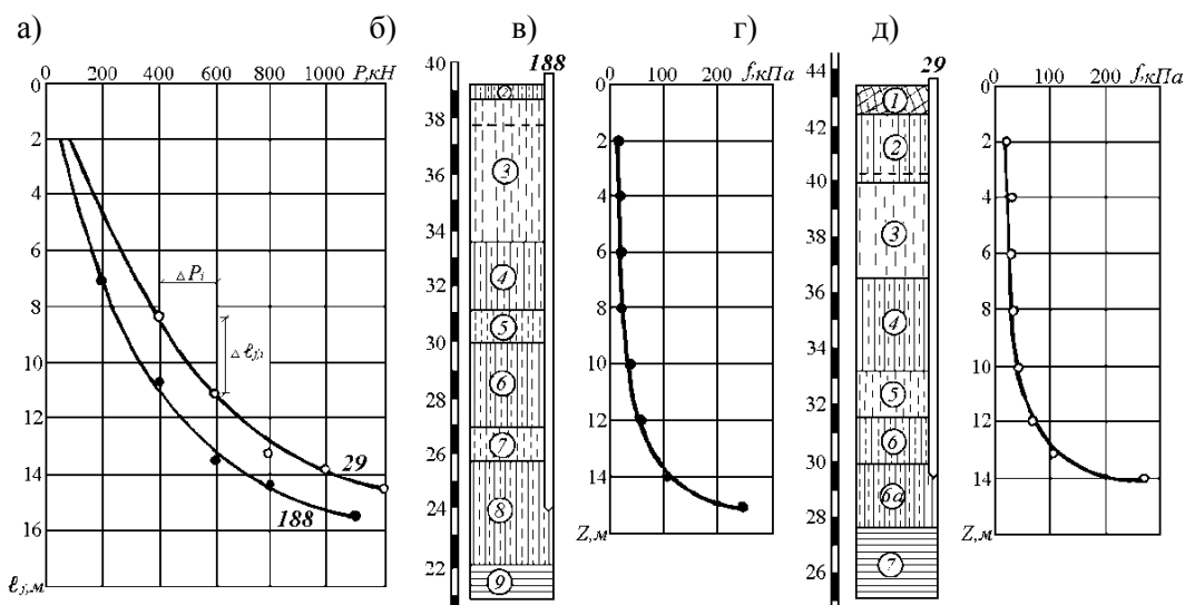
Рис.2. Визначення опору зрушенню по довжині палі: а) графіки залежності довжини пружно-стисненої ділянки стовбура палі від навантаження; б; г) інженерно-геологічна будова ділянок будівництва; в; д) графіки зміни опору зрушенню по глибині для палей №№188 і 29. Пунктирною лінією показано рівень підземних вод
