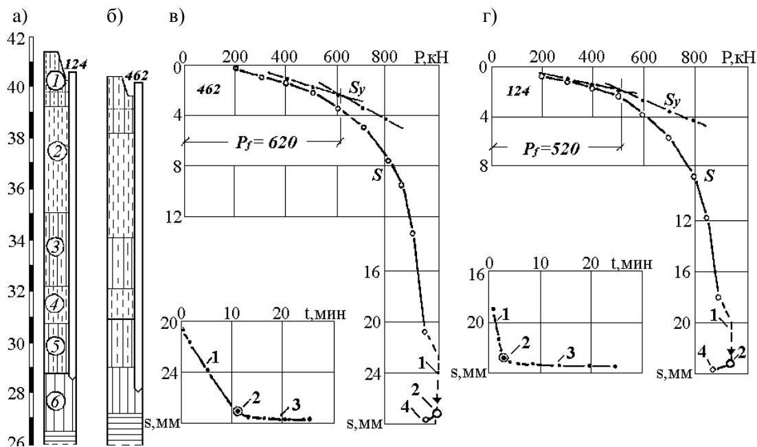
Рис.3. Результати випробувань ґрунтів палями на вертикальне вдавлююче навантаження: а) б) інженерно-геологічні колонки в точці випробувань палі; в) г) графіки залежності осідання від навантаження: 1. «зрив» палі. 2. Припинення підкачки масла в камеру домкрату. 3. Процес зниження навантаження та стабілізації деформацій. 4. Навантаження, рівноважене силами опору ґрунтів
