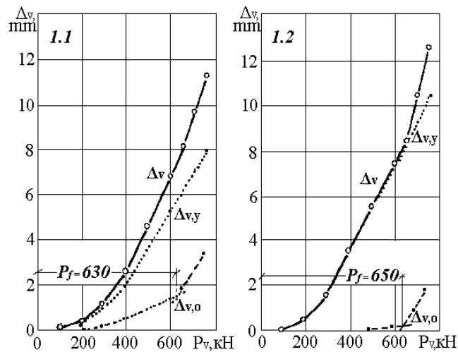
Рис.4. Результати випробувань палі на вертикальне висмикуюче навантаження: 1.1 - перше випробування; 1.2 - повторне
