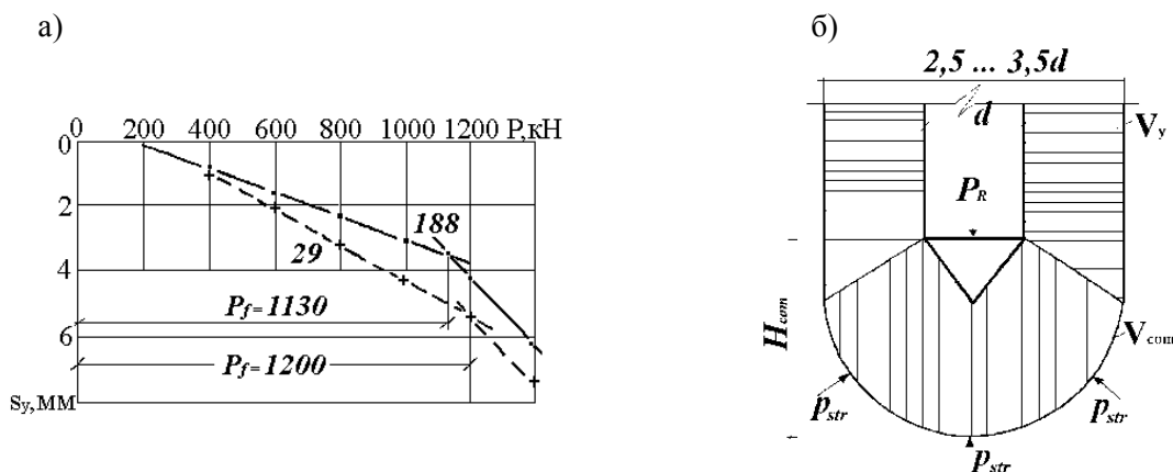
Рис.1. а) графіки залежності пружної складової осідання від навантаження; б) стан ґрунтового середовища після занурення палі: V_y - обсяг ущільненого ґрунту навколо стовбура палі; V_{com} - ущільнене ґрунтове ядро під вістрям палі
