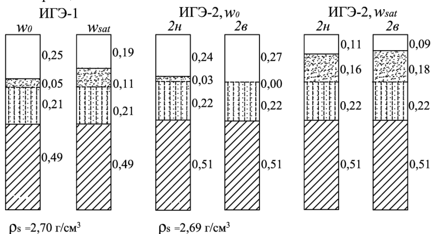
Рисунок 4 – Изменение емкостей фаз и фазовых компонентов при локальном замачивании грунтов на участке Кирхи в г. Одессе
