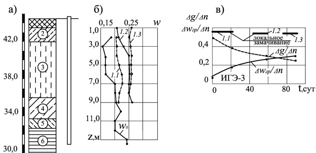
Рисунок 2 – Результаты локального замачивания основания сваи по ул. Парковой в г. Одессе: а) геологическое строение: 2, 4 – суглинки лессовые; 3, 5 - супеси лессовые; 6 – суглинок низкопористый; б) влажность в начале и в процессе каждого этапа замачивания; в) изменение степени заполнения объема пор водой и газом: 1.1, 1.2, 1.3 – обозначение номера испытаний
