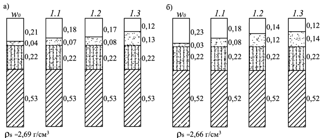
Рисунок 3 – Изменение емкостей фаз и фазовых компонентов при поэтапном локальном замачивании основания свай по ул. Парковой в г. Одессе: а) в пределах ИГЭ-2 ; б) в пределах ИГЭ-3
