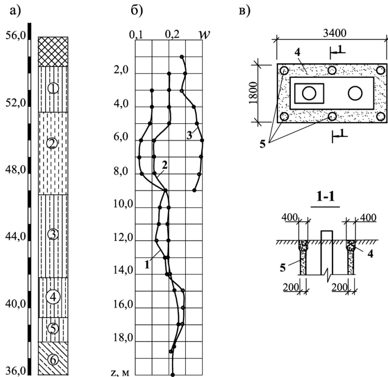
Рисунок 1 – Методика исследований: а) геологическое строение участка застройки Кирхи с линейкой абсолютных отметок; б) влажность по глубине: 1 – при изысканиях, 2 – при проходке скважин для свай, 3 – перед окончанием локального замачивания; в) схема дренажной системы для локального замачивания: 4 – грунтовый лоток, заполненный щебнем; 5 – дренажные скважины, заполненные песком
