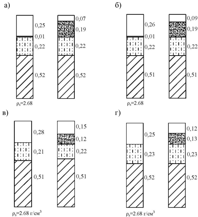
Рисунок 5 – Изменение емкостей фаз и фазовых компонентов при влажности: а, б) капиллярно-поднятой; в, г) капиллярно-подвешенной
