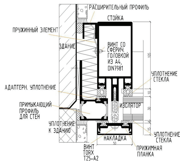
Рисунок 8. Схема бокового примыкания к зданию.
