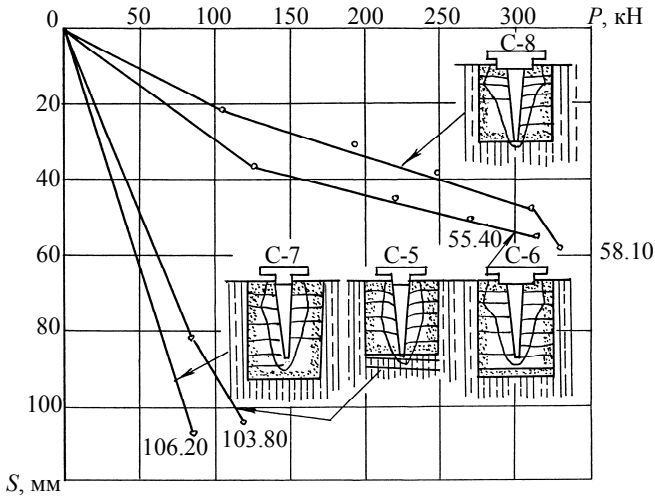
Рисунок 2 – Графики P = f(S) .
