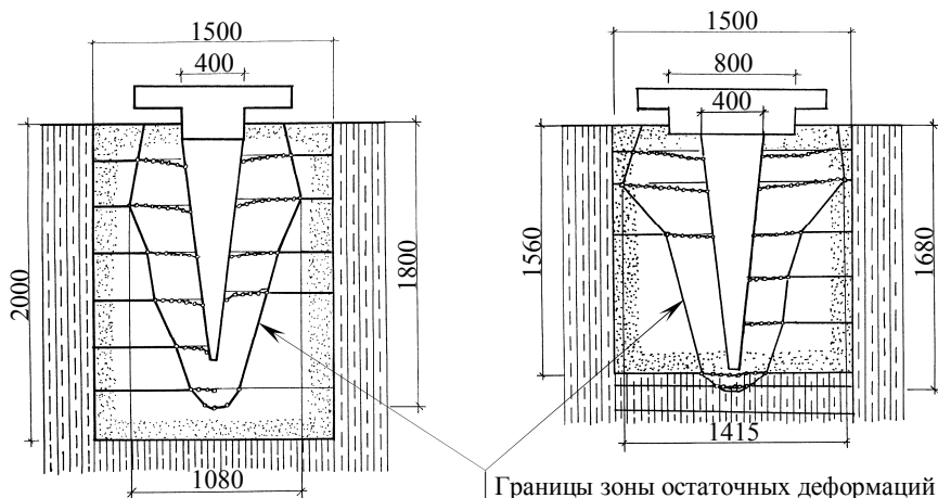
Рисунок 1 – результаты испытаний одиночной сваи С-7 с высоким ростверком и одиночной сваи С-8 с низким ростверком.
