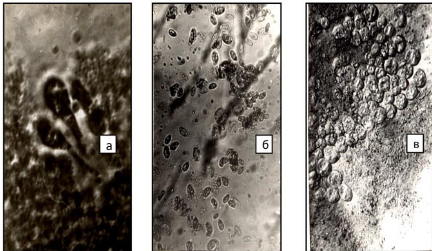
Рис. 1. Микроорганизмы биопленки дисковых биофильтров: а – Vorticella convallaria ; б – Stylonychia pu stulata , Colpoda steine , Paramaecium caudatum ; в – Zooglea ramigera ; г – Nematodes , зооглейные скопления бактерий, ресничные инфузории.
