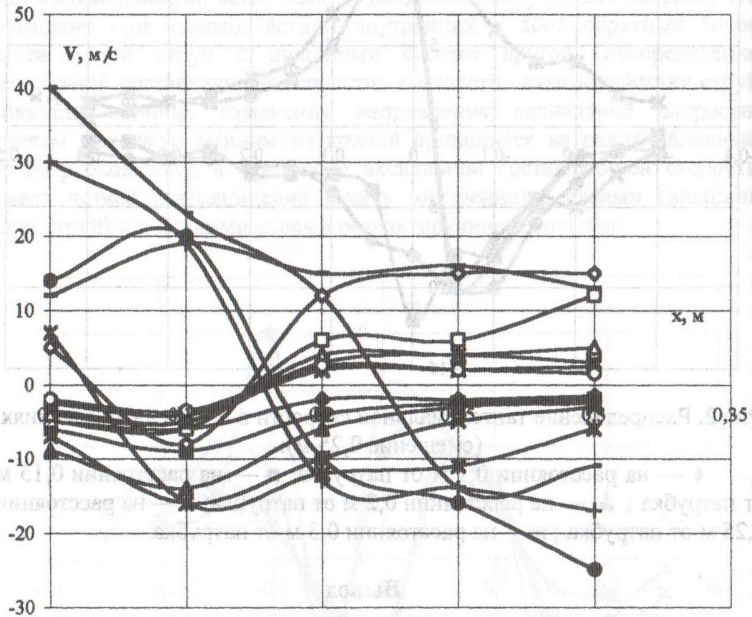
Рис.3. Распределение аксиальной скорости (смещение 0,25 м): ◆ — на расстоянии Z = -0,3 м от оси струи; ■ — на расстоянии Z = -0,25 м от оси струи; ▲ — на расстоянии Z = -0,2 м от оси струи; х — на расстоянии Z = -0,15 м от оси струи; ж — на расстоянии Z = -0,1 м от оси струи; • — на расстоянии Z = -0,05 м от оси струи; + — на оси струи; — — на расстоянии Z = 0,05 м от оси струи; — — на расстоянии Z = 0,1 м от оси струи; ◇ — на расстоянии Z = 0,15 м от оси струи; □ — на расстоянии Z = 0,2 м от оси струи; Δ — на расстоянии Z = 0,25 м от оси струи; — — на расстоянии Z = 0,3 м от оси струи; — — на расстоянии Z = 0,35 м от оси струи; ○ — на расстоянии Z = 0,4 м от оси струи.
