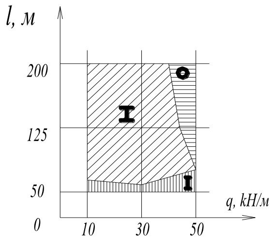
Рис. 5. График для определения рационального типа сечения верхнего пояса в зависимости от пролета и нагрзуки
