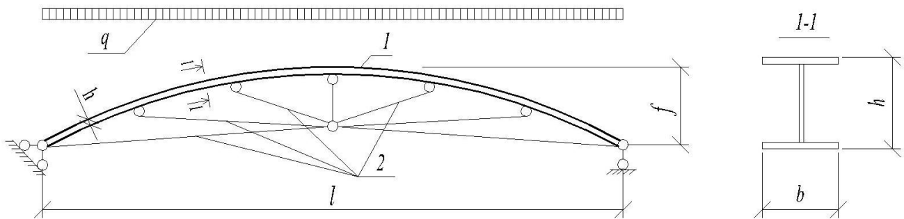
Рис. 1. Схема конструкции ( f/l = const = 1/6 ) 1 – жесткий верхний пояс; 2 – элементы гибкой решетки
