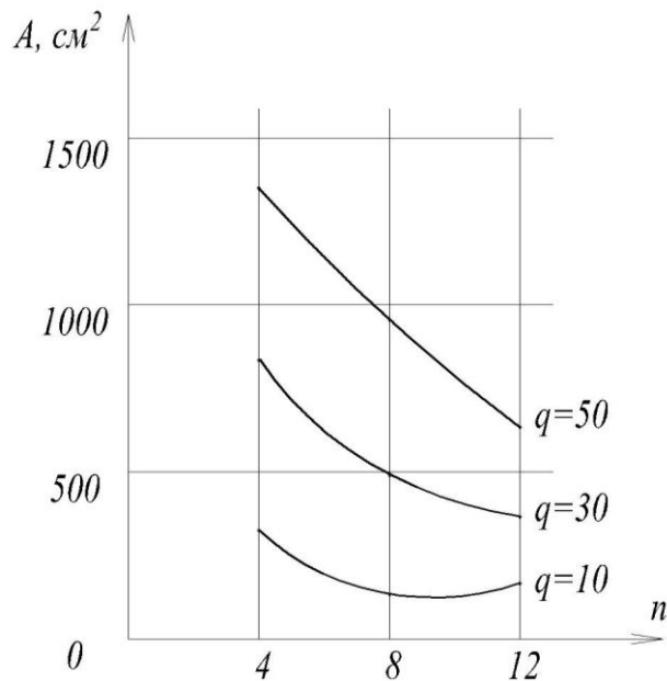
Рис. 3. Зміна площі сечення верхнього пояса в залежності від кількості панелей верхнього пояса при пролеті l = 125 м
