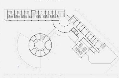
План на відм +4.500 М 1:200
